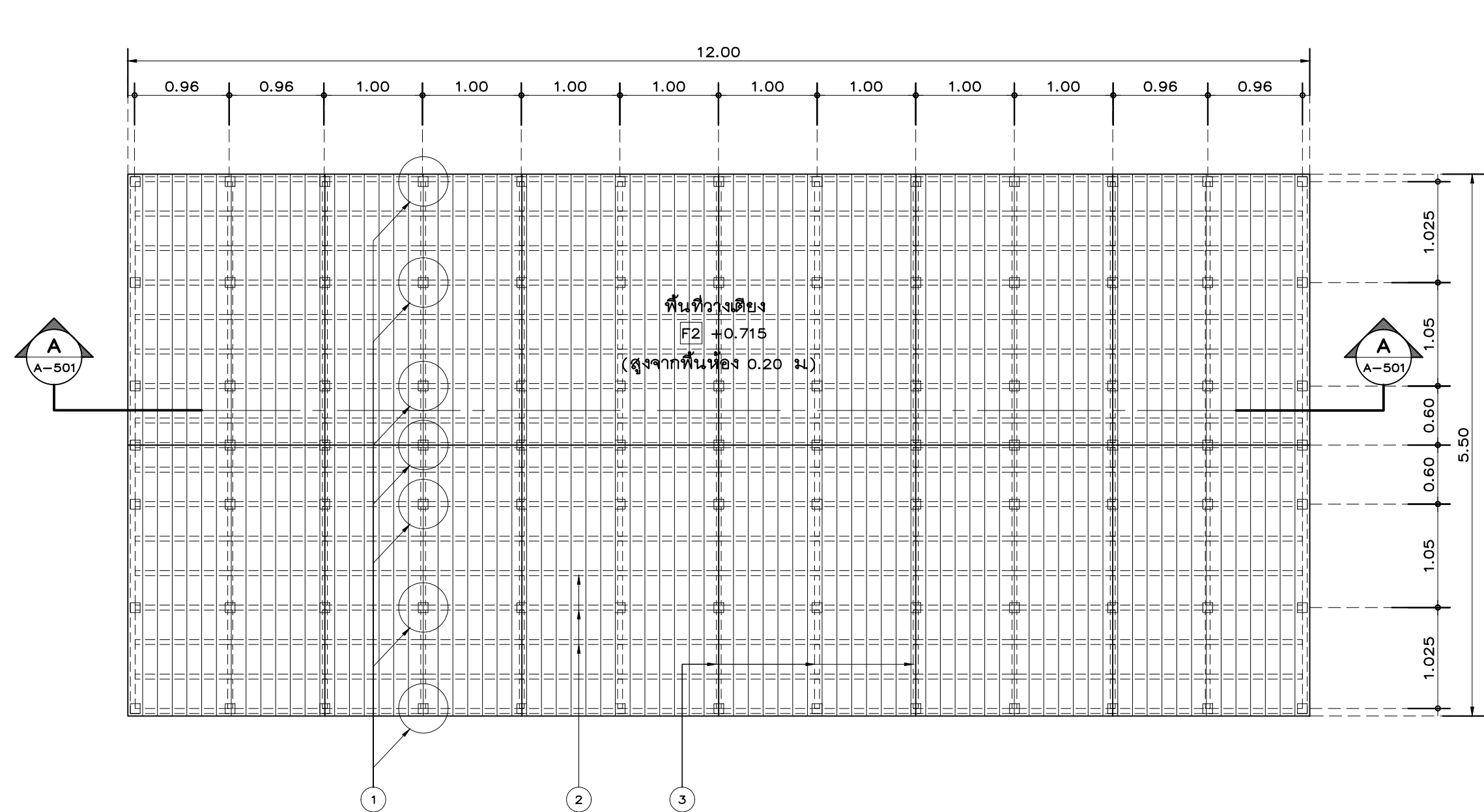
แปลน มาตราส่วน 1: 50
