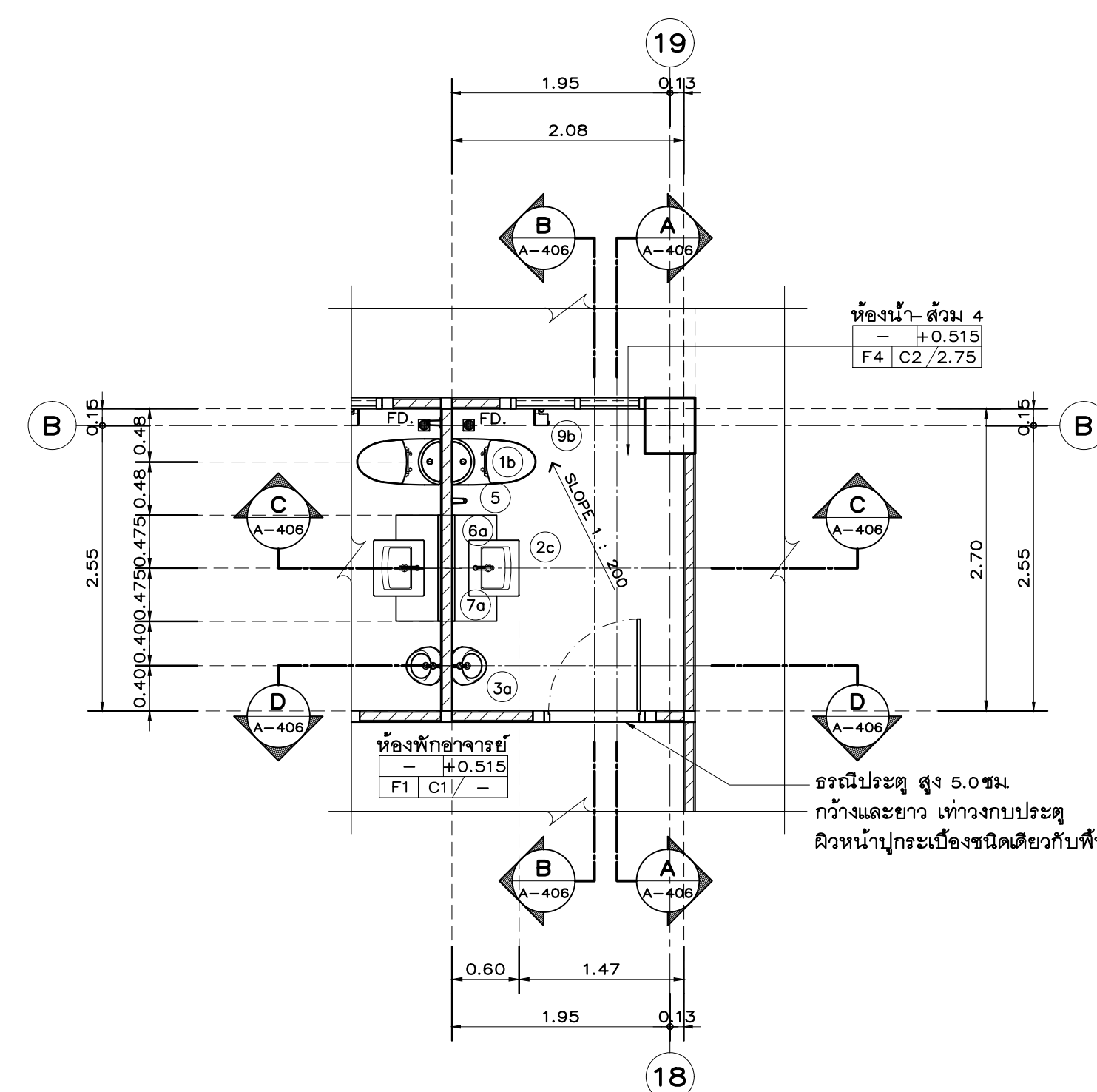
แปลนพื้นห้องน้ำ – ส่วน 4
