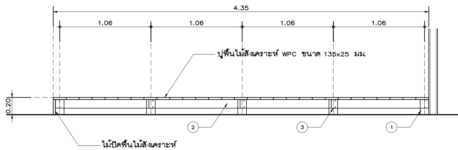
รูปตัด C-C มาตราส่วน 1: 25
