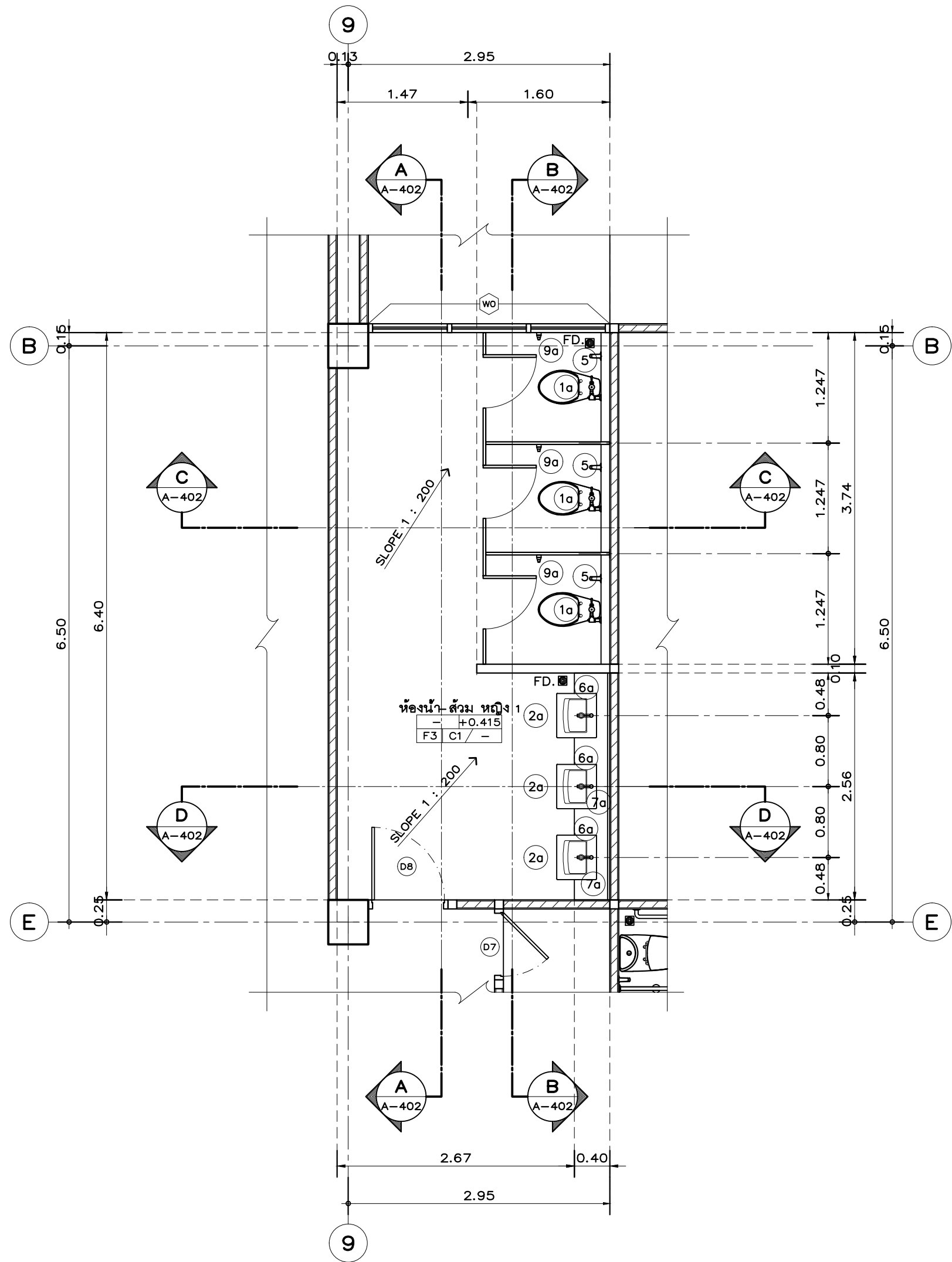
แปลนพื้นห้องน้ำ – ส้วม หญิง 1 มาตราส่วน 1: 50
