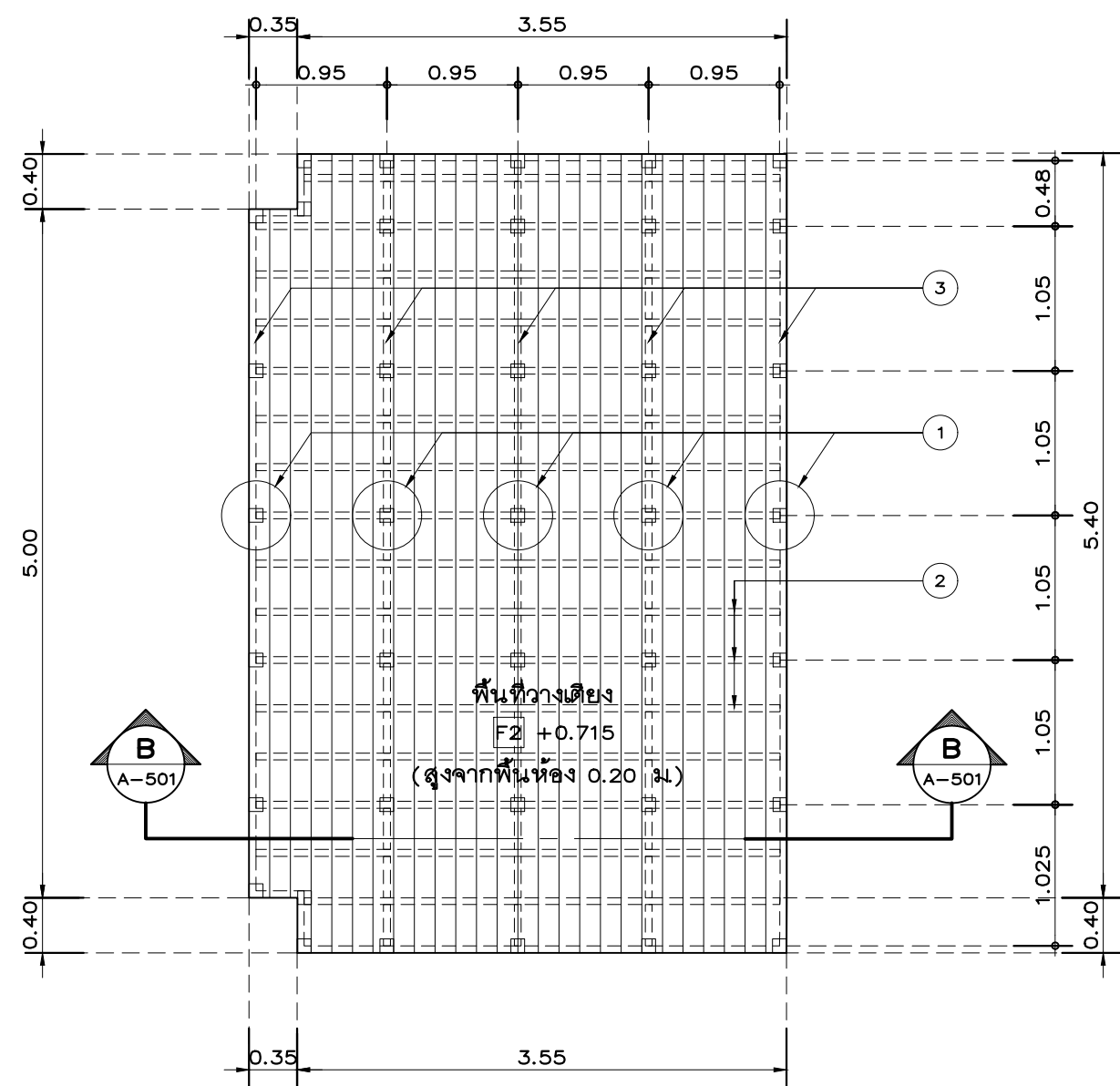
แปลน มาตราส่วน 1: 50
