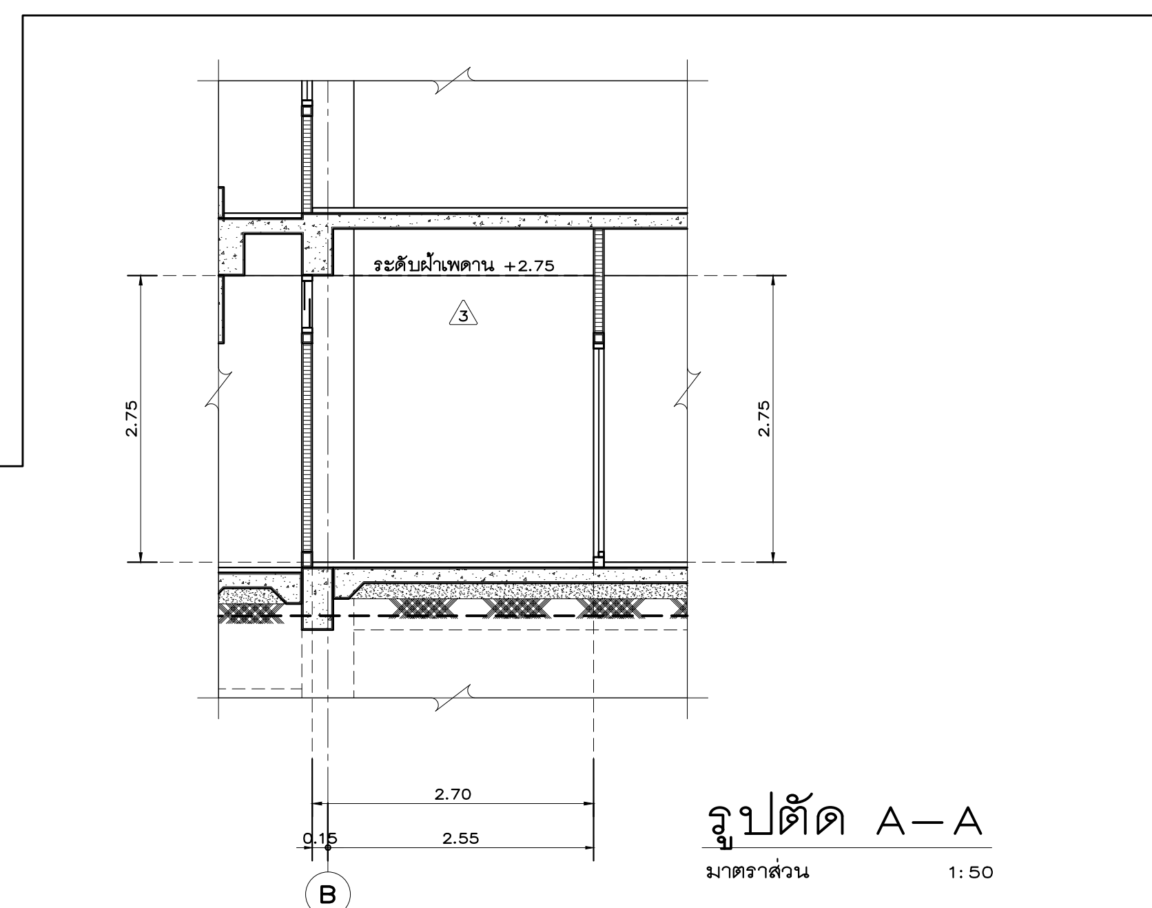
รูปตัด A-A
