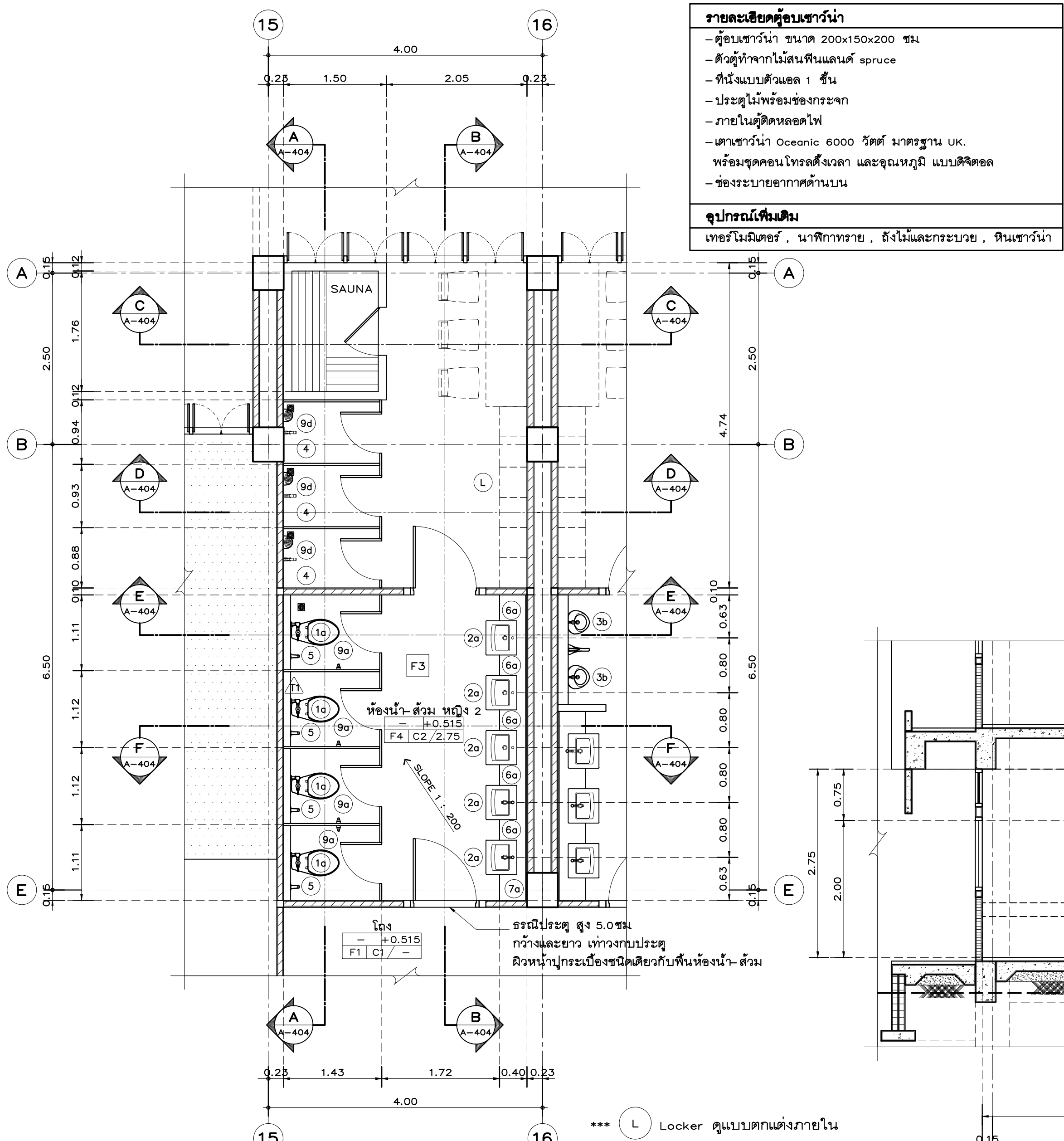
แปลนพื้นห้องน้ำ - ส่วน หญิง 2
