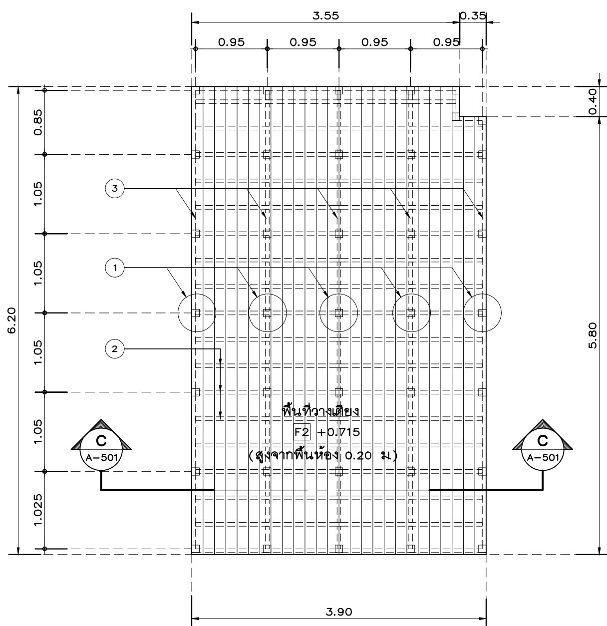
แปลน มาตราส่วน 1: 50
