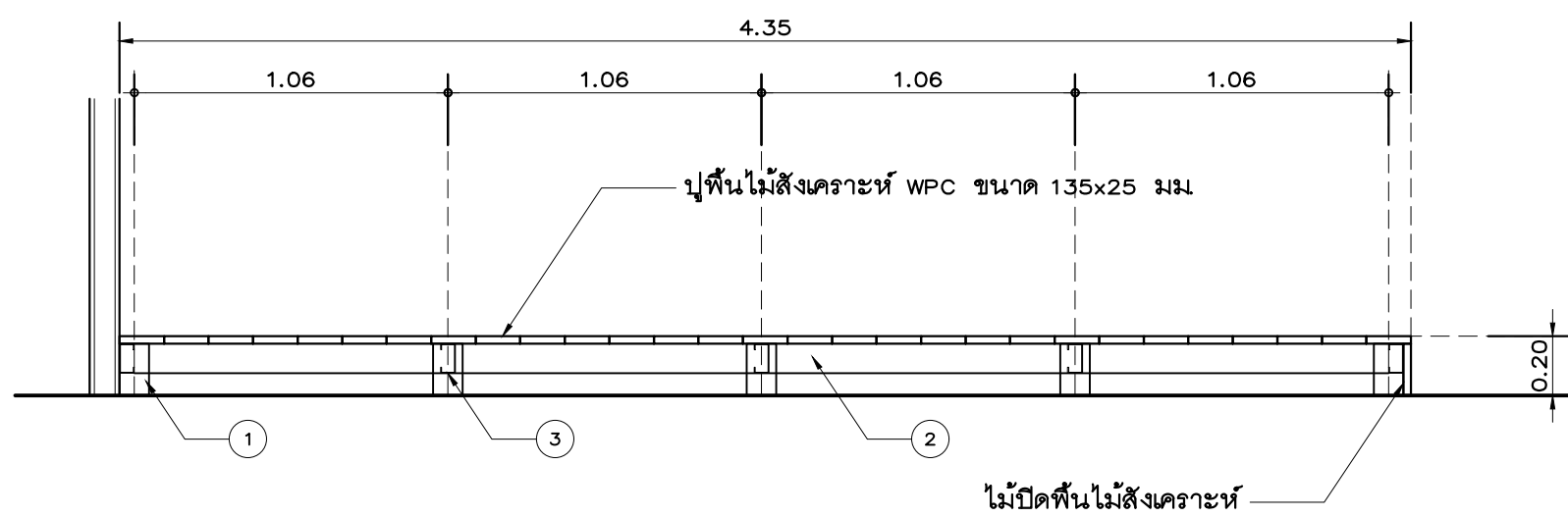
รูปตัด B-B มาตราส่วน 1: 25
