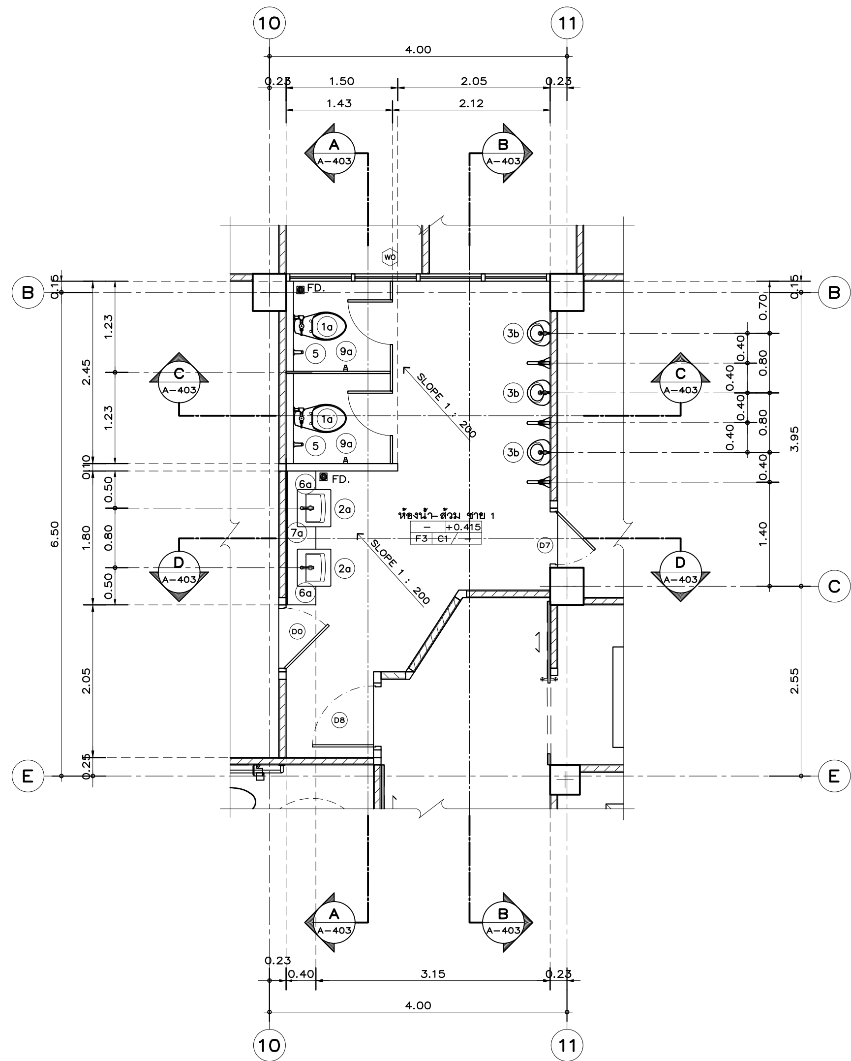
แปลนพื้นห้องน้ำ – ส้วม ซ้าย 1 มาตรฐาน 1: 50
