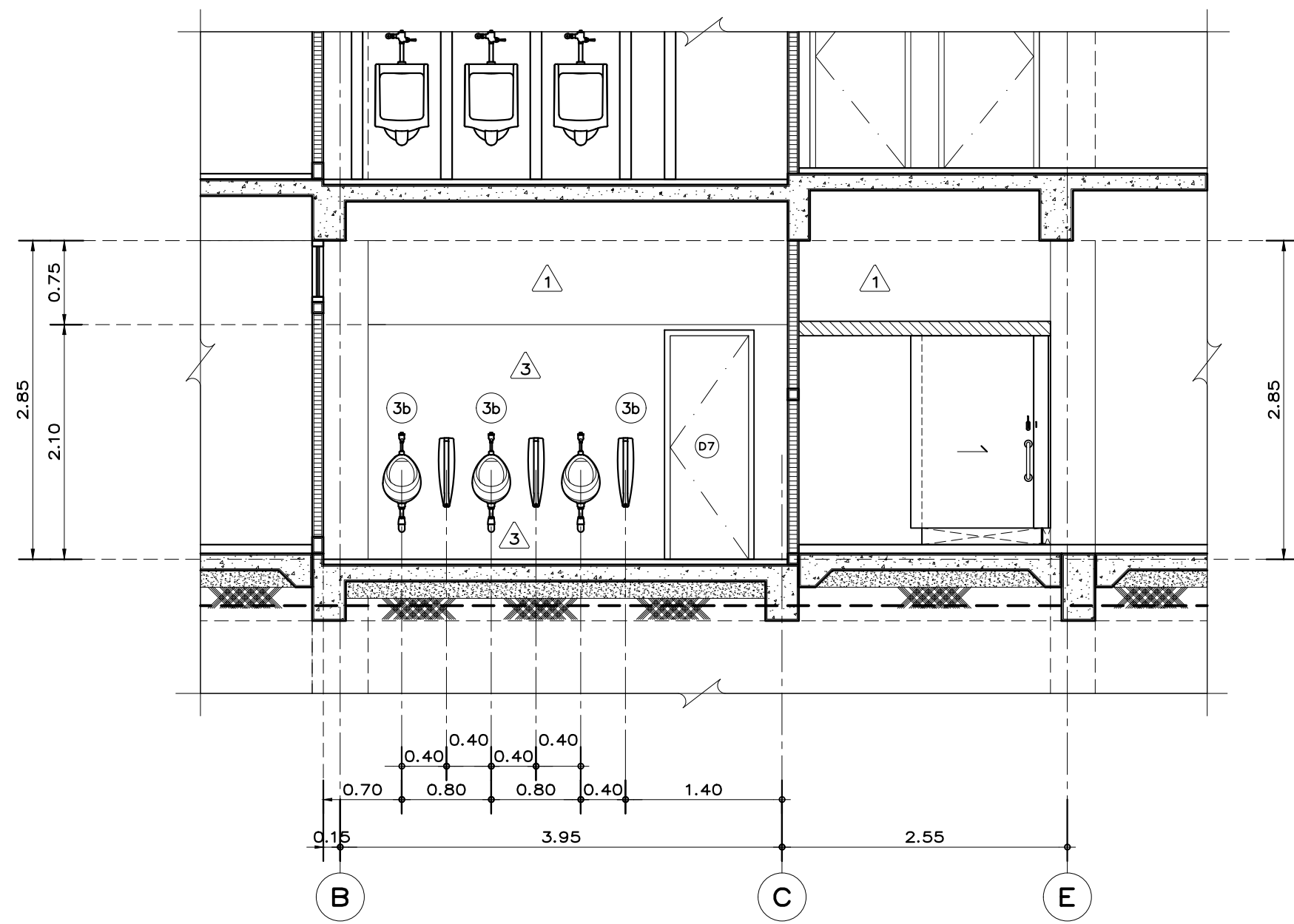
รูปตัด B-B มาตรฐาน 1: 50
